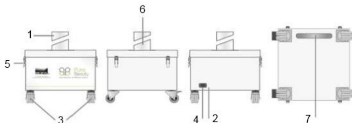
Внешний вид дымоуловителя Salon Guard
